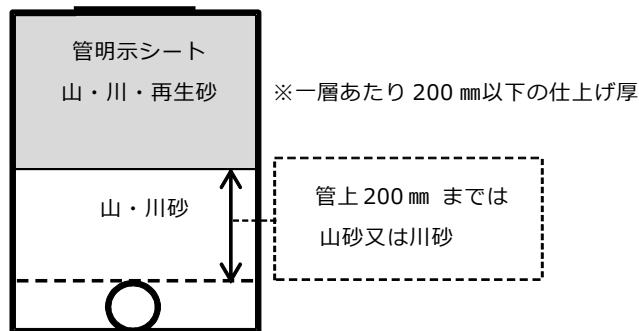
図 9-1…埋戻し工事概略図
